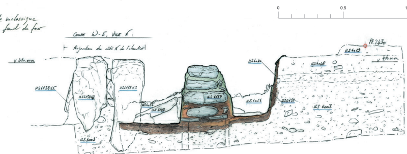
Dessin de terrain représentant l'un des fours de potier de Vufflens, en plan et en coupe. Dessin A. Pignolet, Archeodunum.
