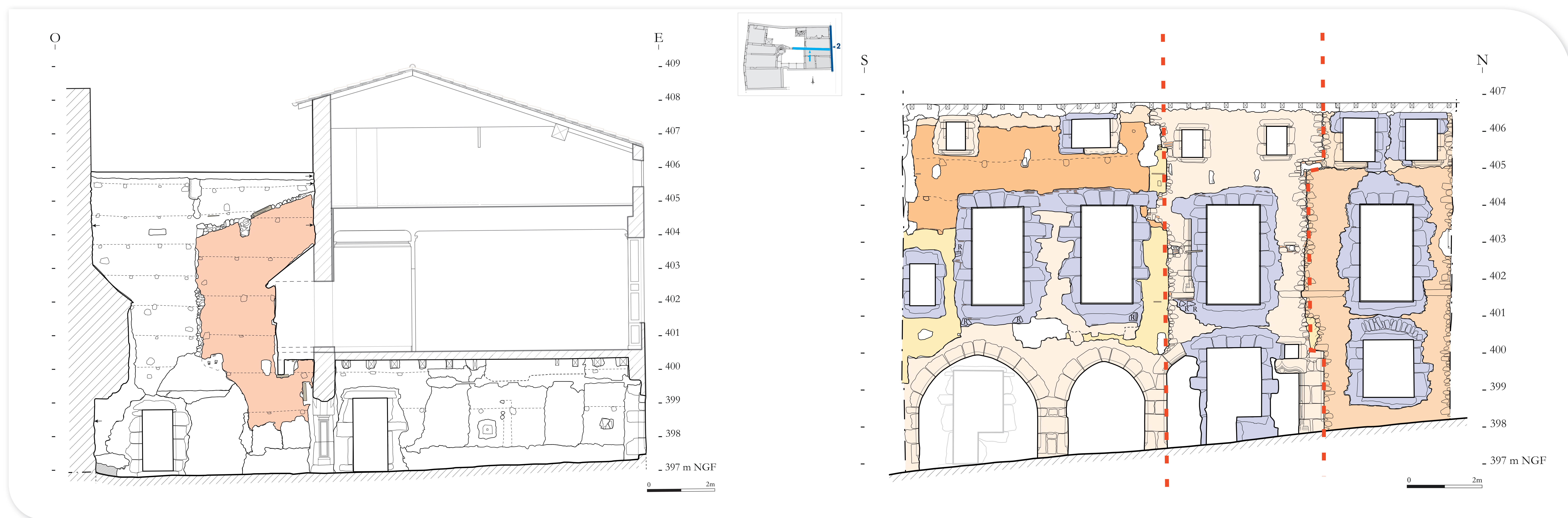
1. Relevé d'élévation à l'intérieur de l'îlot. La partie colorée correspond au bâtiment initial. - 2. Relevé de la façade orientale
