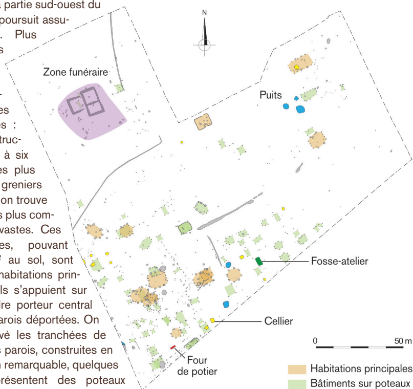
Fig.2 : Plan des vestiges archéologiques.
